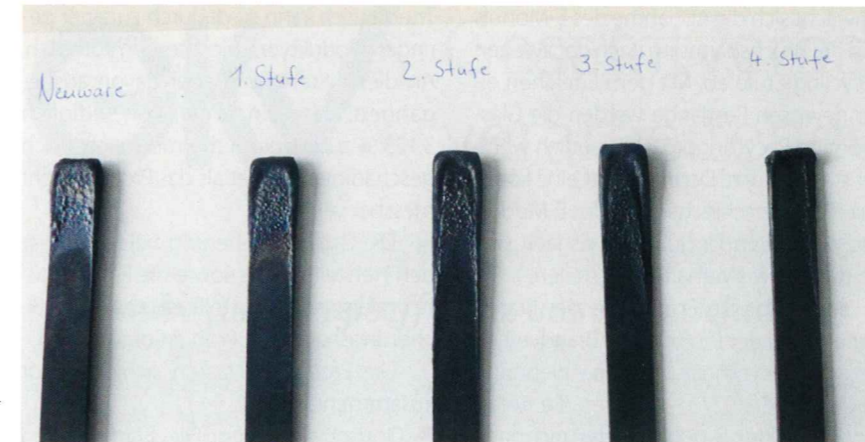
Bild 2. Ergebnisse der Brandprüfungen: Die flammhemmende Wirkung des roten Phosphors wird durch den Recyclingprozess nicht beeinträchtigt © Ostfalia Hochschule für angewandte Wissenschaften
